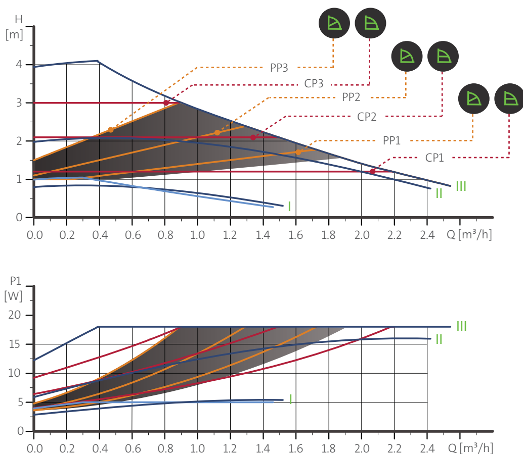
Abb. 30 ALPHA2 XX-40
