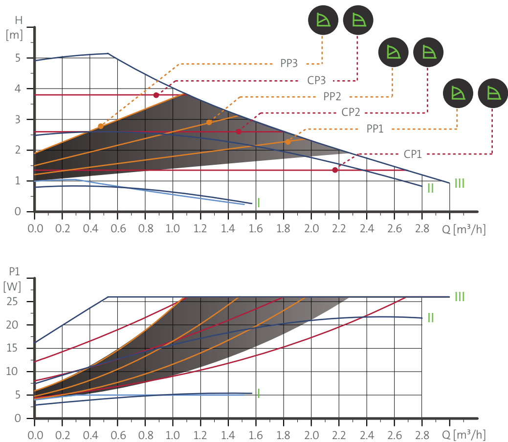
Abb. 31 ALPHA2 XX-50
