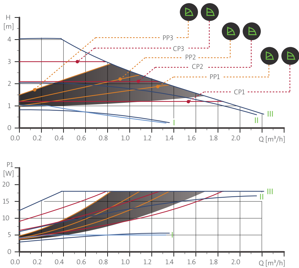
Abb. 33 ALPHA2 25-40 A
