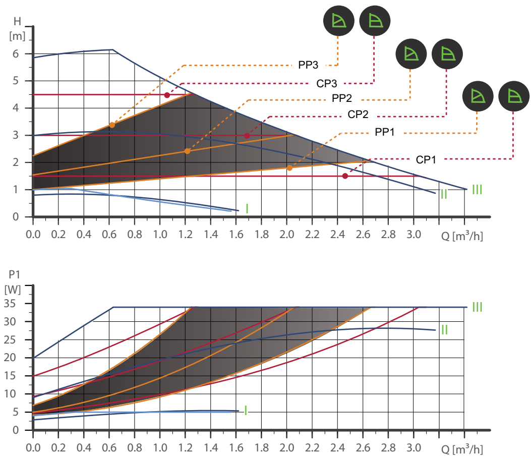
Abb. 32 ALPHA2 XX-60
